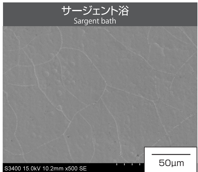
めっき皮膜の表面SEM像 SEM image (surface)
